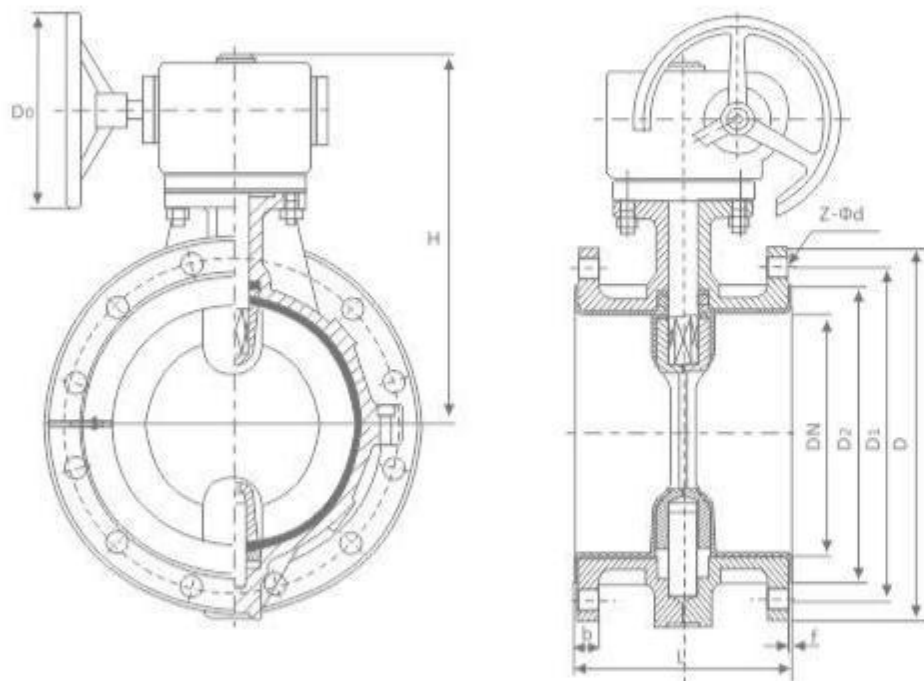
DA341 F/P 型法兰连接蜗轮传动蝶阀（中线） DA341 F/P Worm drive flanged butterfly valve (middle)
